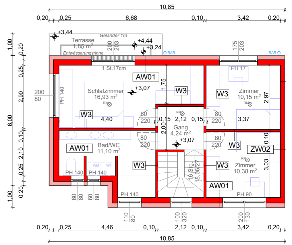
GRUNDRISS OBERGESCHOSS 1:100
