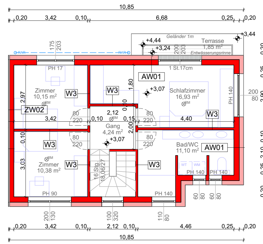
GRUNDRISS OBERGESCHOSS 1:100
