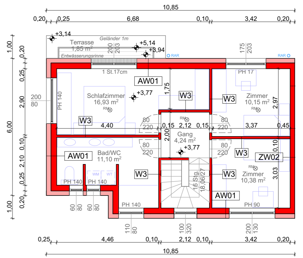
GRUNDRISS OBERGESCHOSS 1:100
