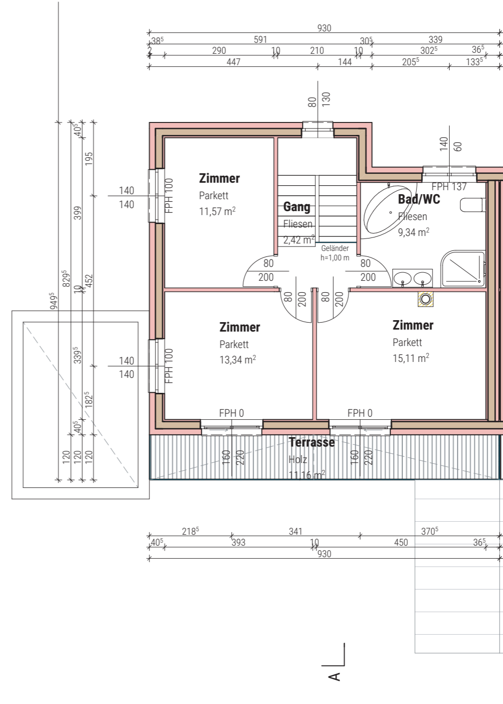
1. OG 1:100
