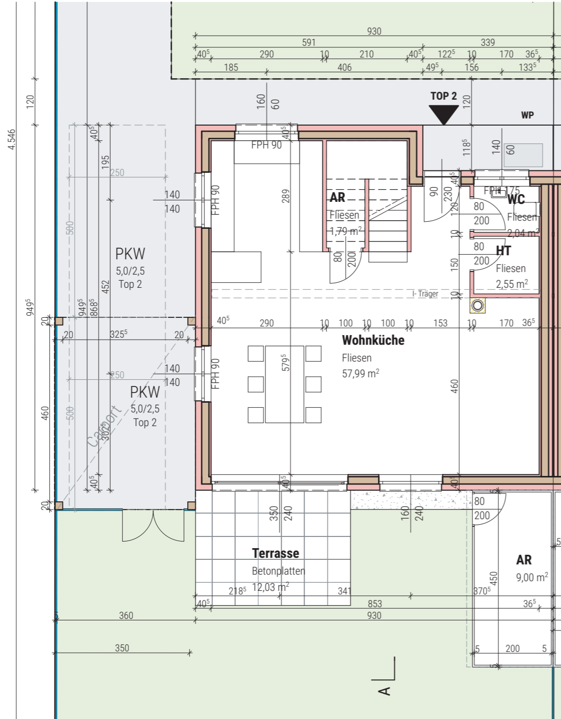
0. EG 1:100
