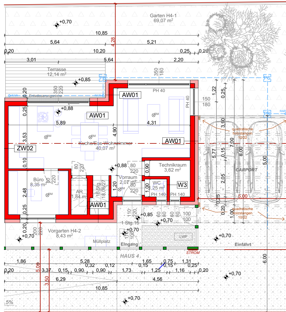
GRUNDRISS ERDGESCHOSS Haus 4 - TYP 2
