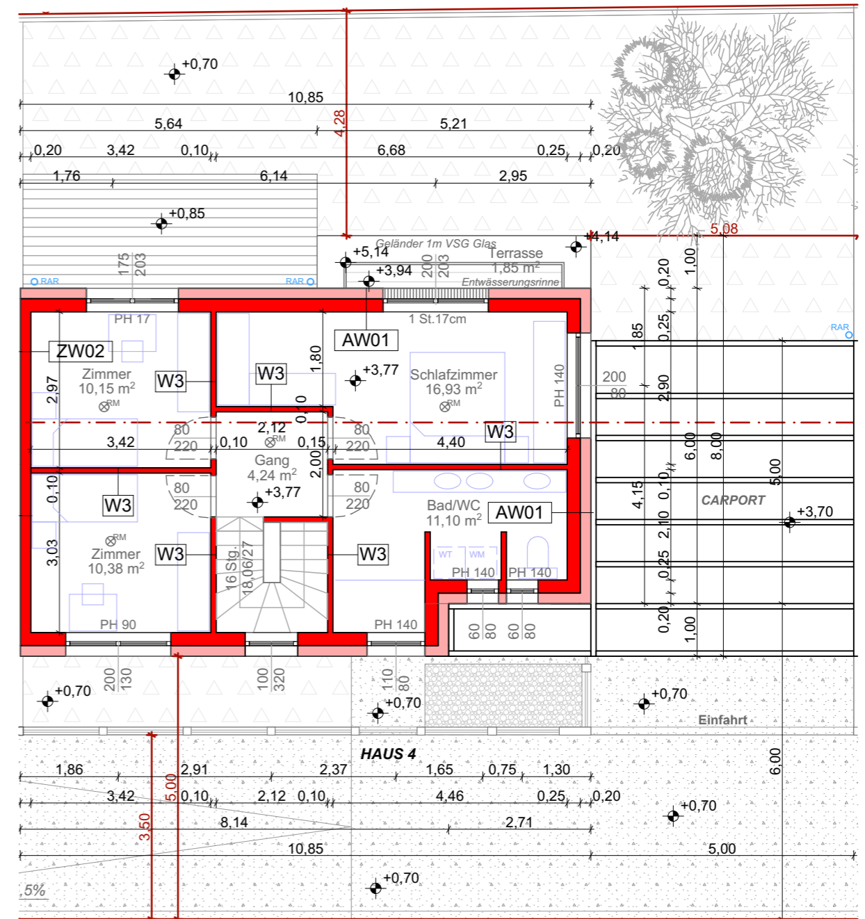
GRUNDRISS OBERGESCHOSS Haus 4 - TYP 1 und TYP 2
