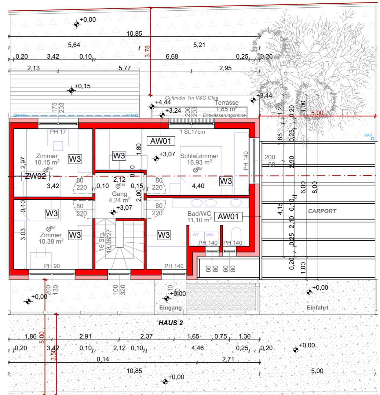
GRUNDRISS OBERGESCHOSS Haus 2 - TYP 1 und TYP 2
