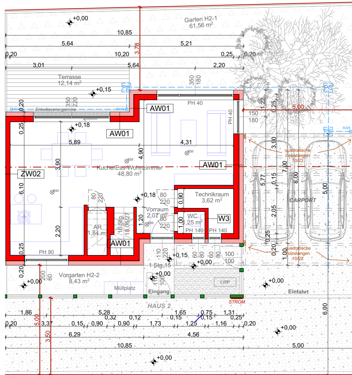
GRUNDRISS ERDGESCHOSS Haus 2 - TYP 1
